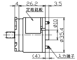
TP-3526A・B・C-HM・PHM
