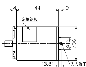
TP-3644D・H-HM・PHM
