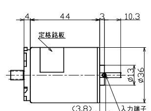
TP-3644J・L-HM・PHM
