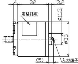
TP-3644D・H-HM・PHM
