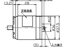
TP-3644J・L-HM・PHM
